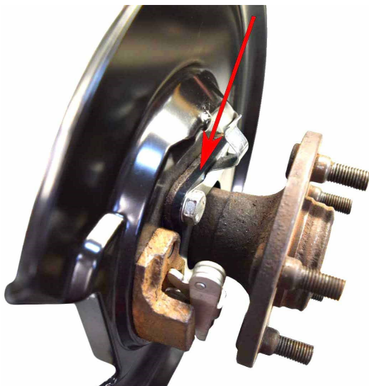
Förstärkningsplåt / Reinforcement Plate
